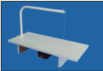
Mesa de Corte Standard 30 cm Medidas: 670 mm x 295 mm, altura 300 mm CÓD. PRODUTO: 1546
