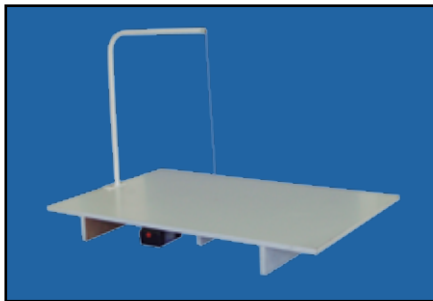
Mesa de Corte Profissional GG Medidas: 1100 mm x 700 mm, alt 600 mm CÓD. PRODUTO: 4976
